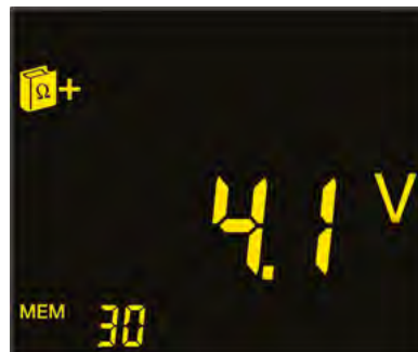
2. Anzeige: Berührungsspannung
